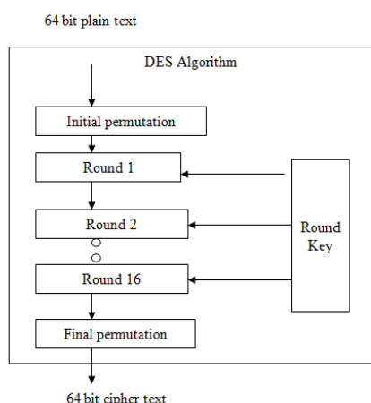
Fig 7 DES
