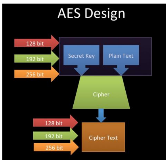
Fig 8 AES
